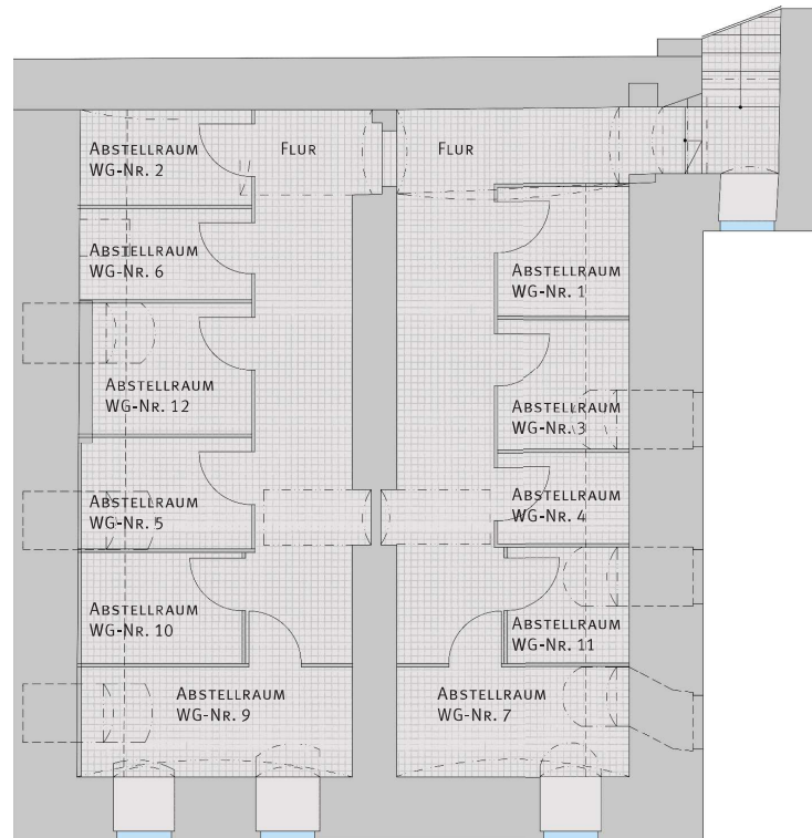
Kellergeschoss
