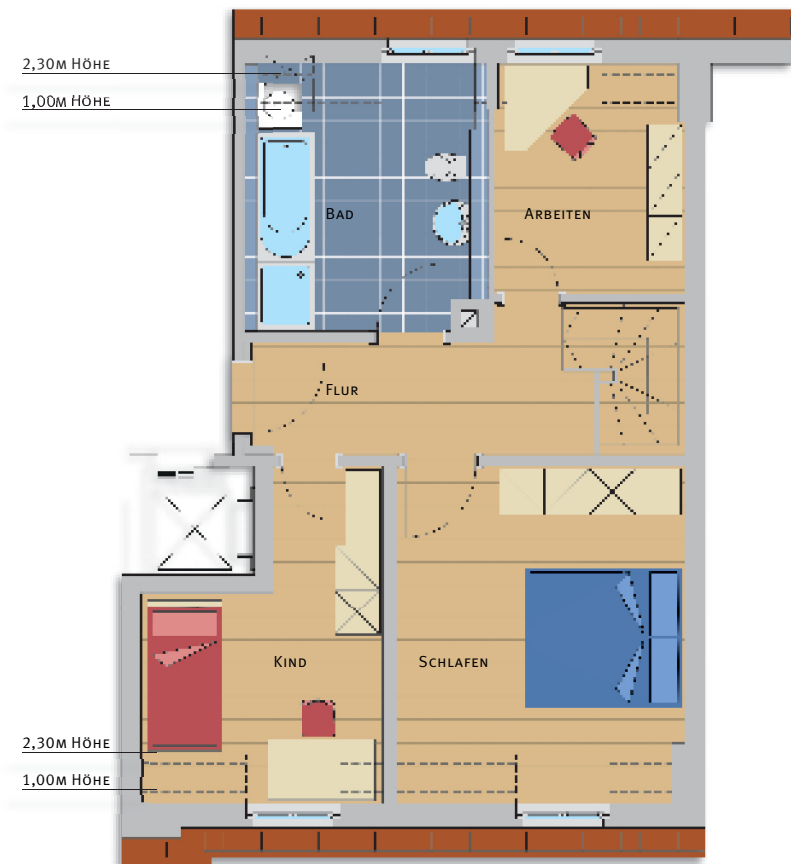
MANSARDENGESCHOSS
