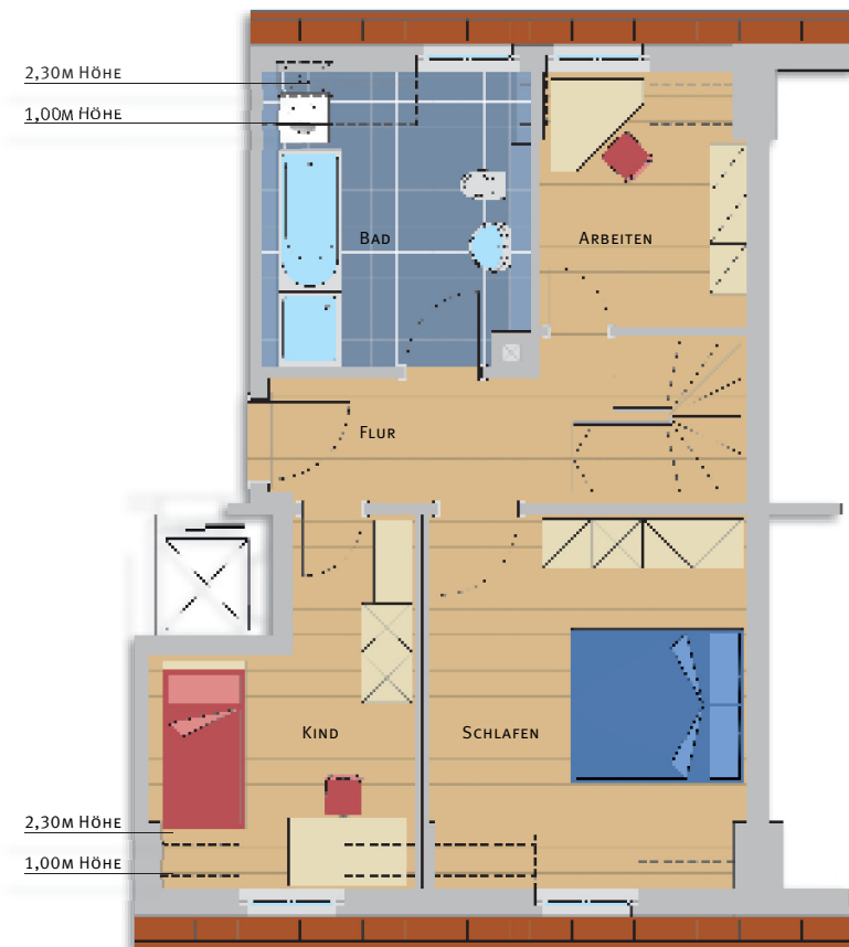
MANSARDENGESCHOSS
