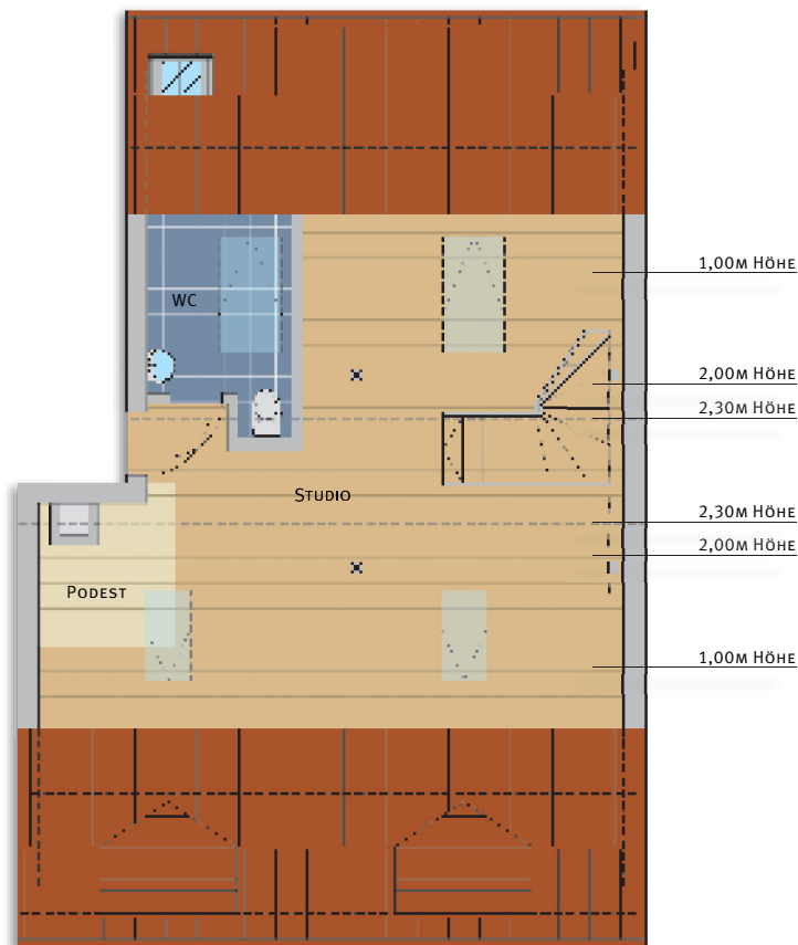
DACHGESCHOSS
